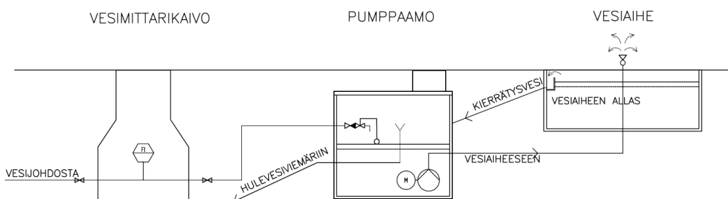
Vesiaiheen periaatekaavio
