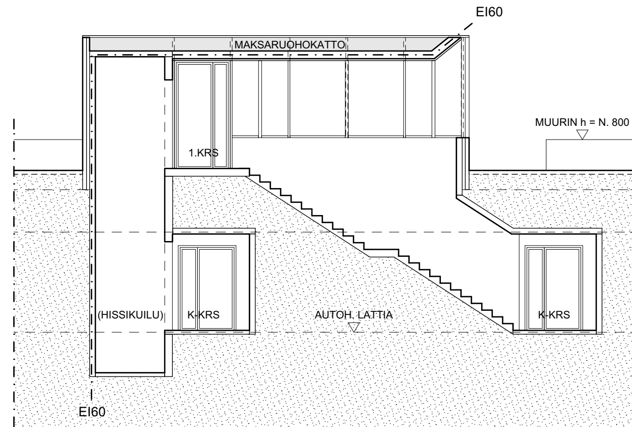
LEIKKAUS 1-1
