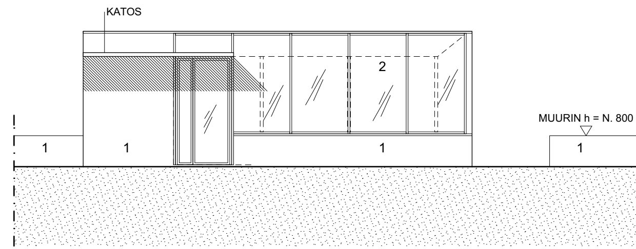
JULKISIVU PIHALLE
