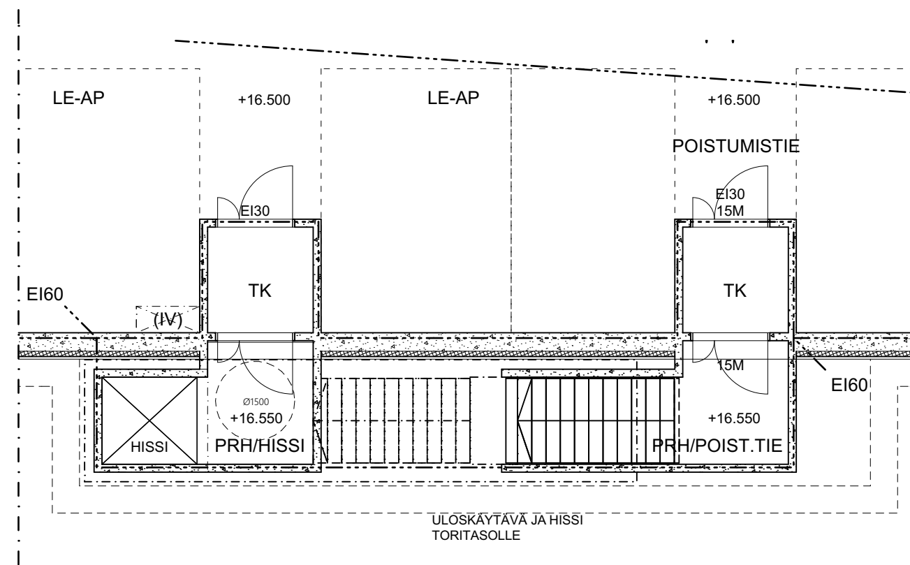
POHJA, KELLARIKERROS
