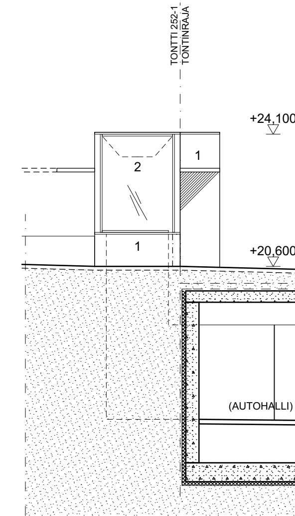
PÄÄTY ITÄÄN
